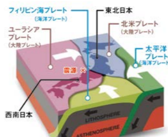
日本列島周辺のプレートの配置 出典：弘前大学大学院公表資料より
